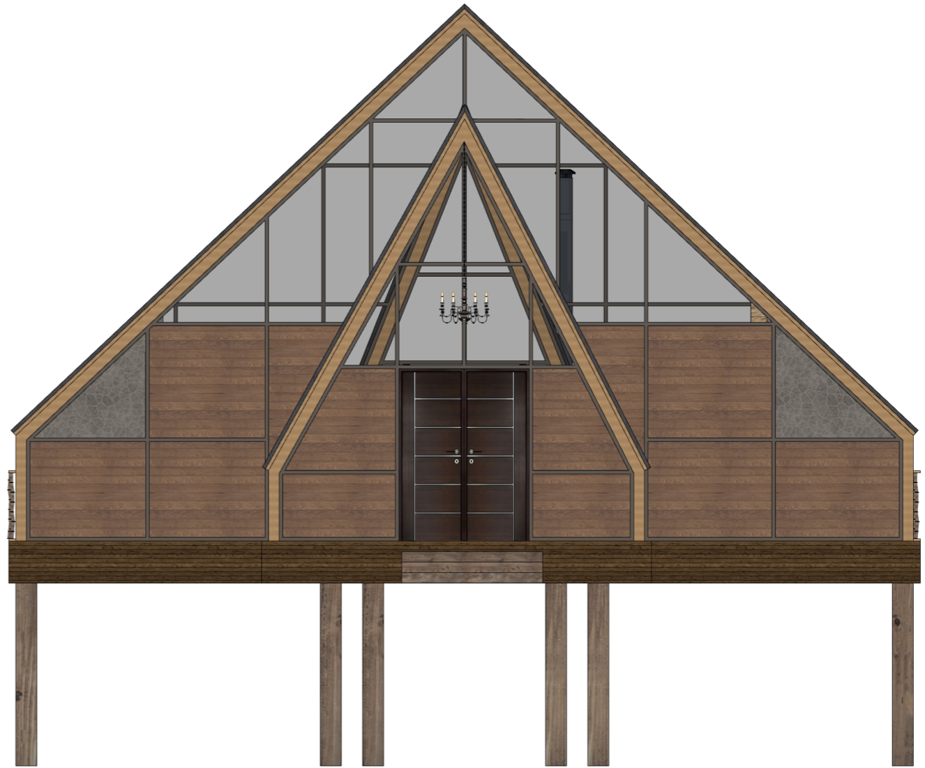
F.E FRONT ELEVATION A00 Scale: 1 mm:75 mm
