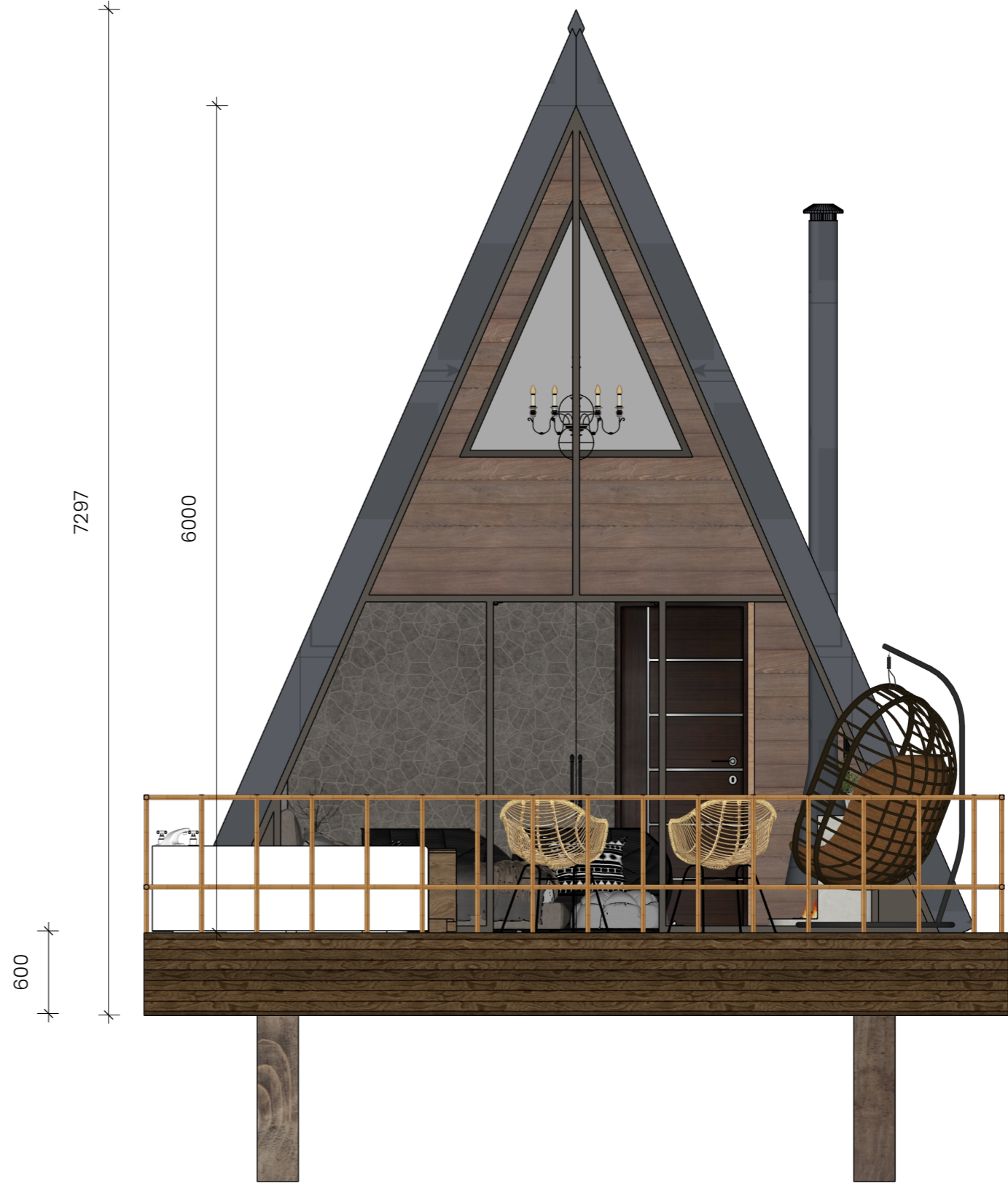
B.E BACK ELEVATION A00 Scale: 1 mm:40 mm
