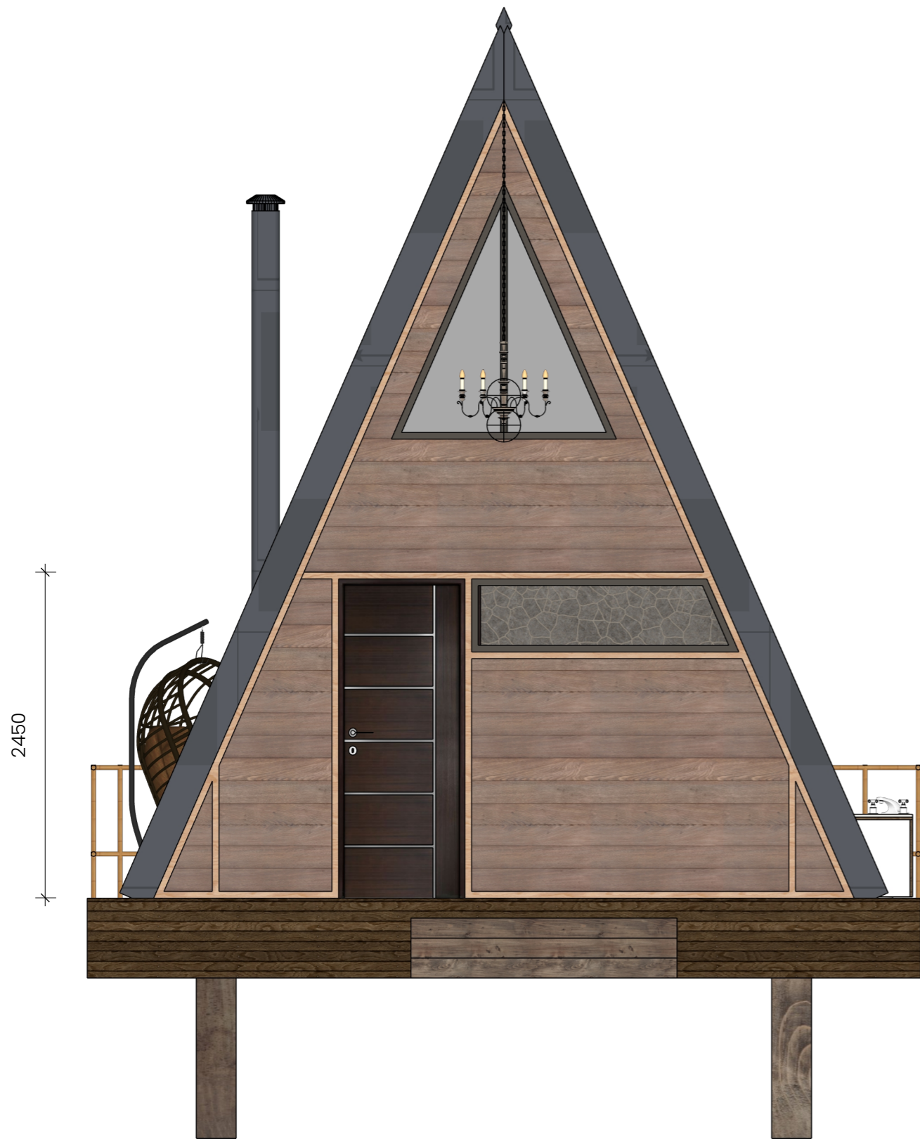
F.E FRONT ELEVATION A01 Scale: 1 mm:40 mm
