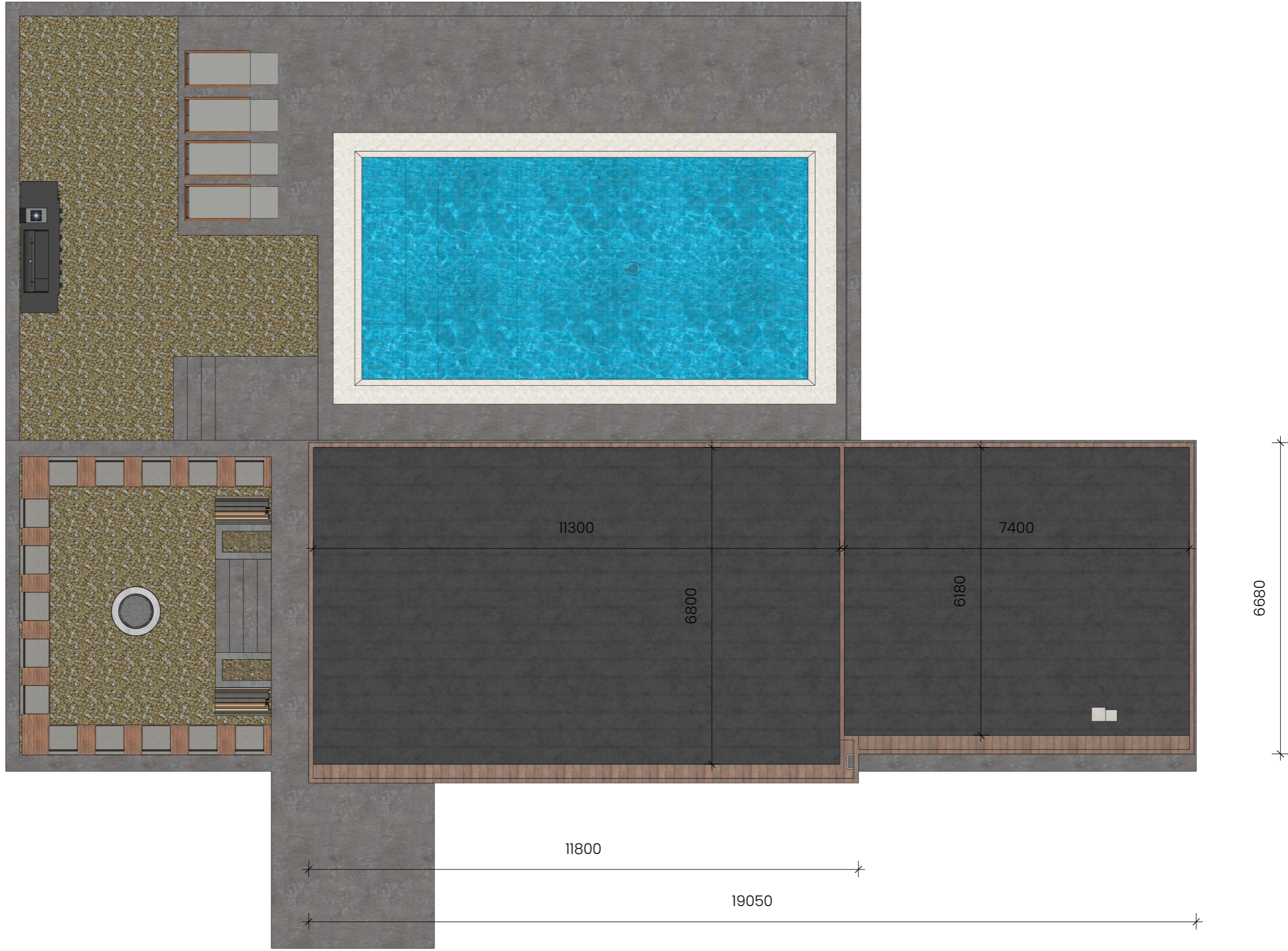
F.P R ROOF PLAN A00 Scale: 1 mm:90 mm
