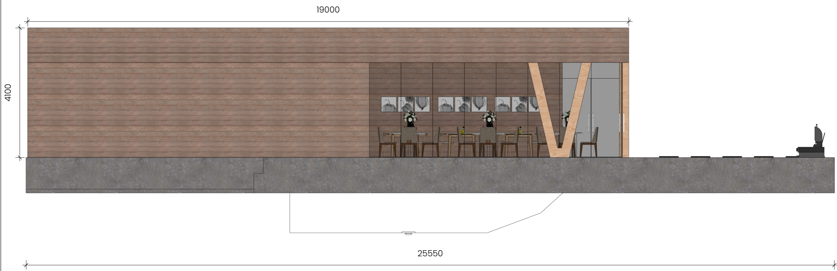
L.E LEFT ELEVATION A01 Scale: 1 mm:75 mm
